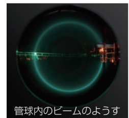
管球内のビームのようす
