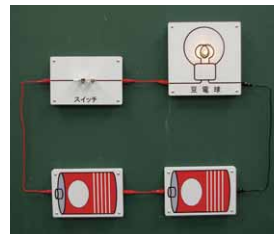
▲乾電池の直列実験
